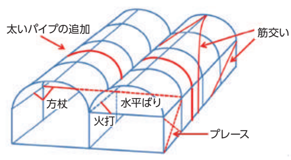
図 ハウスの補強例
