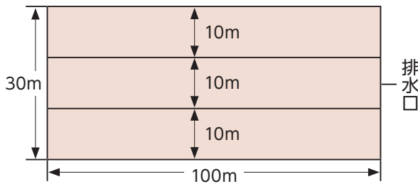
図 30a ほ場の排水溝(明渠)の例
